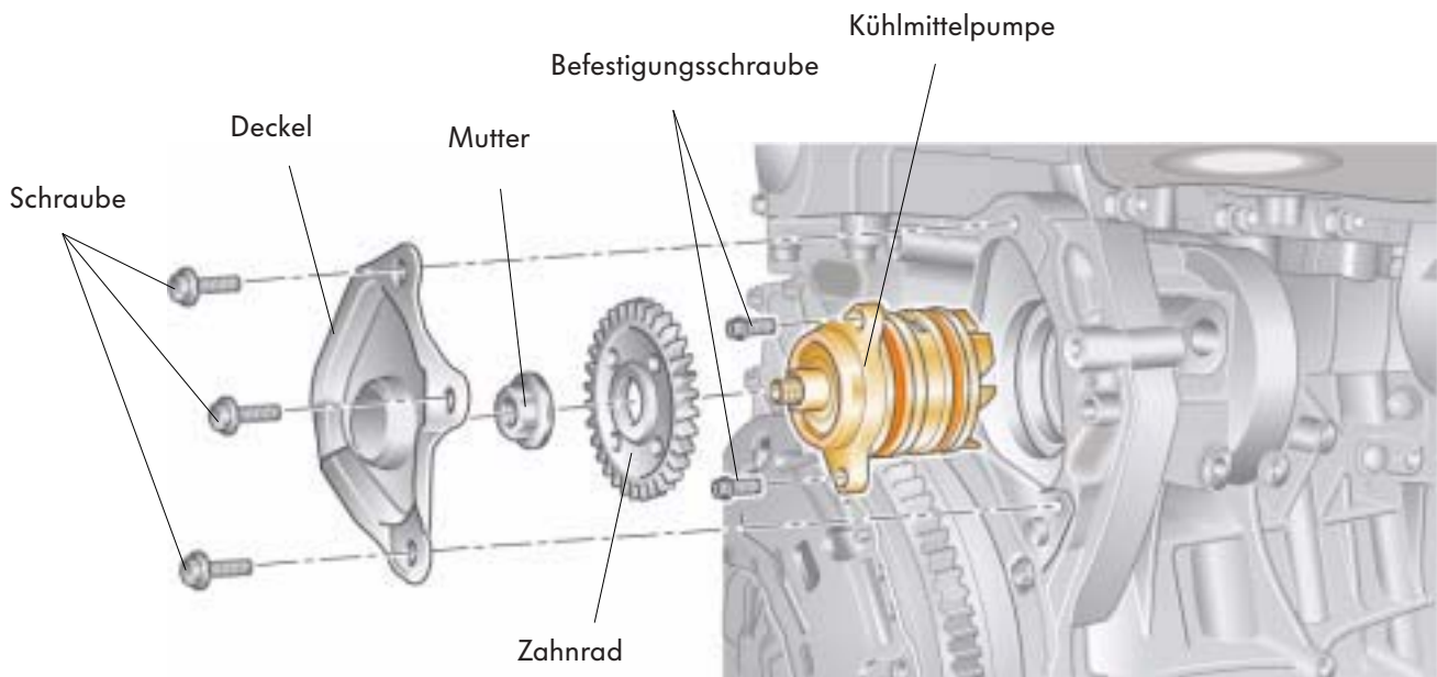
305_050 Kühlmittelpumpe Befestigungsschraube Deckel Mutter Zahnrad Schraube
