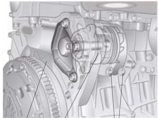
305_049 Steuergehäuse Kühlmittelpumpe Kühlmittelablassschraube
